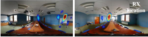
Figure 11. Répartition spatiale de l'énergie ( \tau=9ns )
