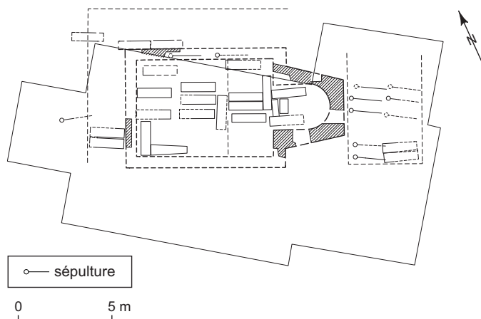
Fig. 44 – Plan de l'église primitive de Meinier (Genève), VI e -VII e s. (DAO : Service cantonal d'archéologie de Genève).
