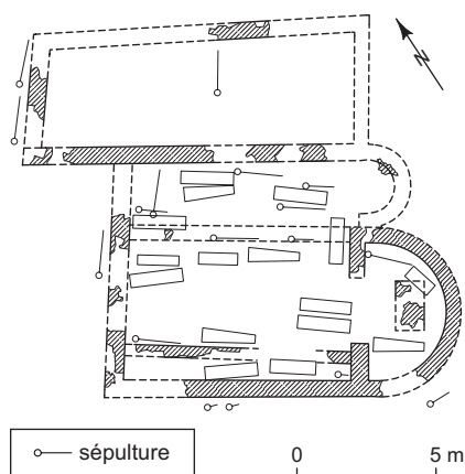
Fig. 43 – Plan de l'église primitive de Saint-Julien-en-Genevois (Haute-Savoie), V e s. (DAO : Service cantonal d'archéologie de Genève).
