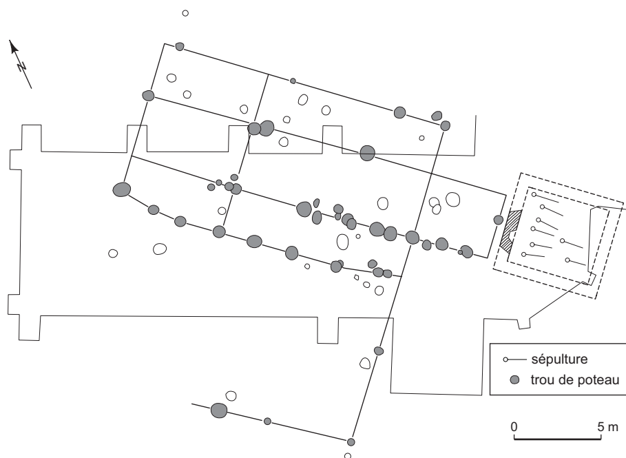
Fig. 47 – Plan de l'église primitive de Satigny (Genève), VIII e -IX e s. (DAO : Service cantonal d'archéologie de Genève).
