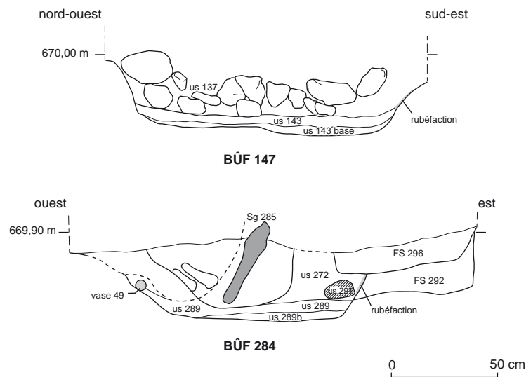
Fig. 119 – Chape de blocs sur le bûcher 147 du Replat à Aime, Savoie (relevé : F. Blaizot, Inrap ; DAO : V. Bastard, Inrap).
