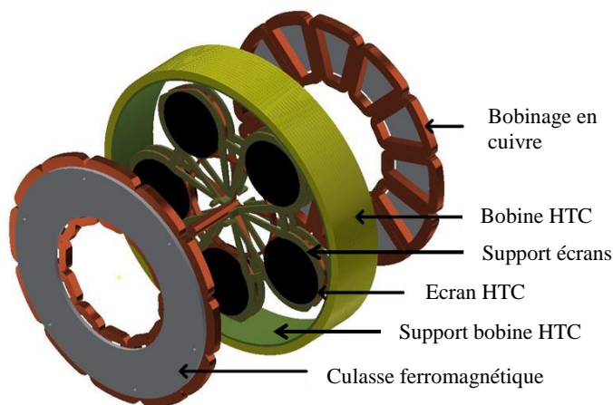
Fig. 1. Vue des éléments actifs de la machine électrique
