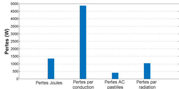
Fig. 4. Répartition des pertes de la machine supraconductrice
