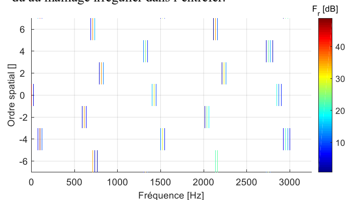
Figure 14 : FFT2D de la pression radiale obtenue par la méthode des sous-domaines.
