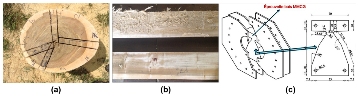
Fig. 1 : (a) Lieu de prélèvements des échantillons du bois vert sur la grume; (b) Poutrelles extraites ; (c) Essais mécaniques via l'éprouvette MMCG
