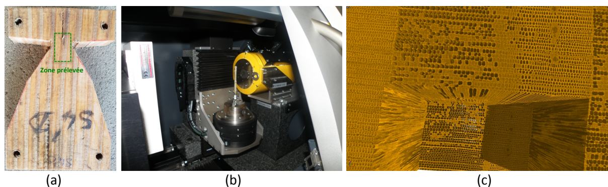
Fig. 2 : (a) Eprouvette en bois de sapin ; (b) Microtomographe à Rayons X ; (c) Volume 3D de la région d'intérêt et traitement d'image (Dalla-Salda et al. 2015).
