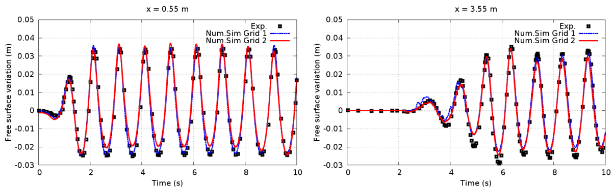
FIGURE 4 – Evolution de la surface libre sur x = 0.55m et x = 3.55m .
