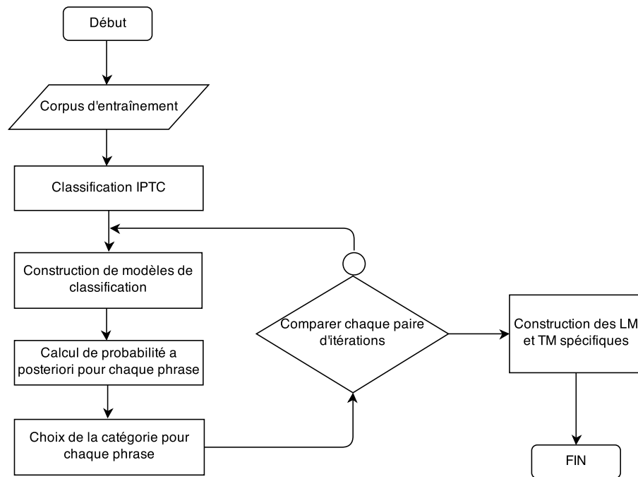
FIG. 2 – Processus itératif pour la construction du classifieur automatique.
