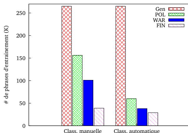
FIG. 3 – Nombre de phrases d’entraînement par catégorie pour les deux scénarios : classification manuelle et automatique.
