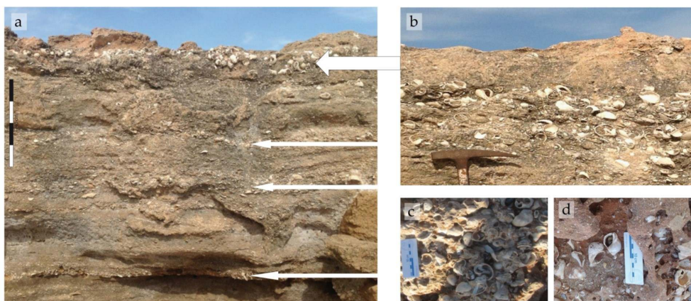
Figure 4 : Dépôts naturels de la région de Rabat-Témara (Carrière 10) riches en coquillages marins.
