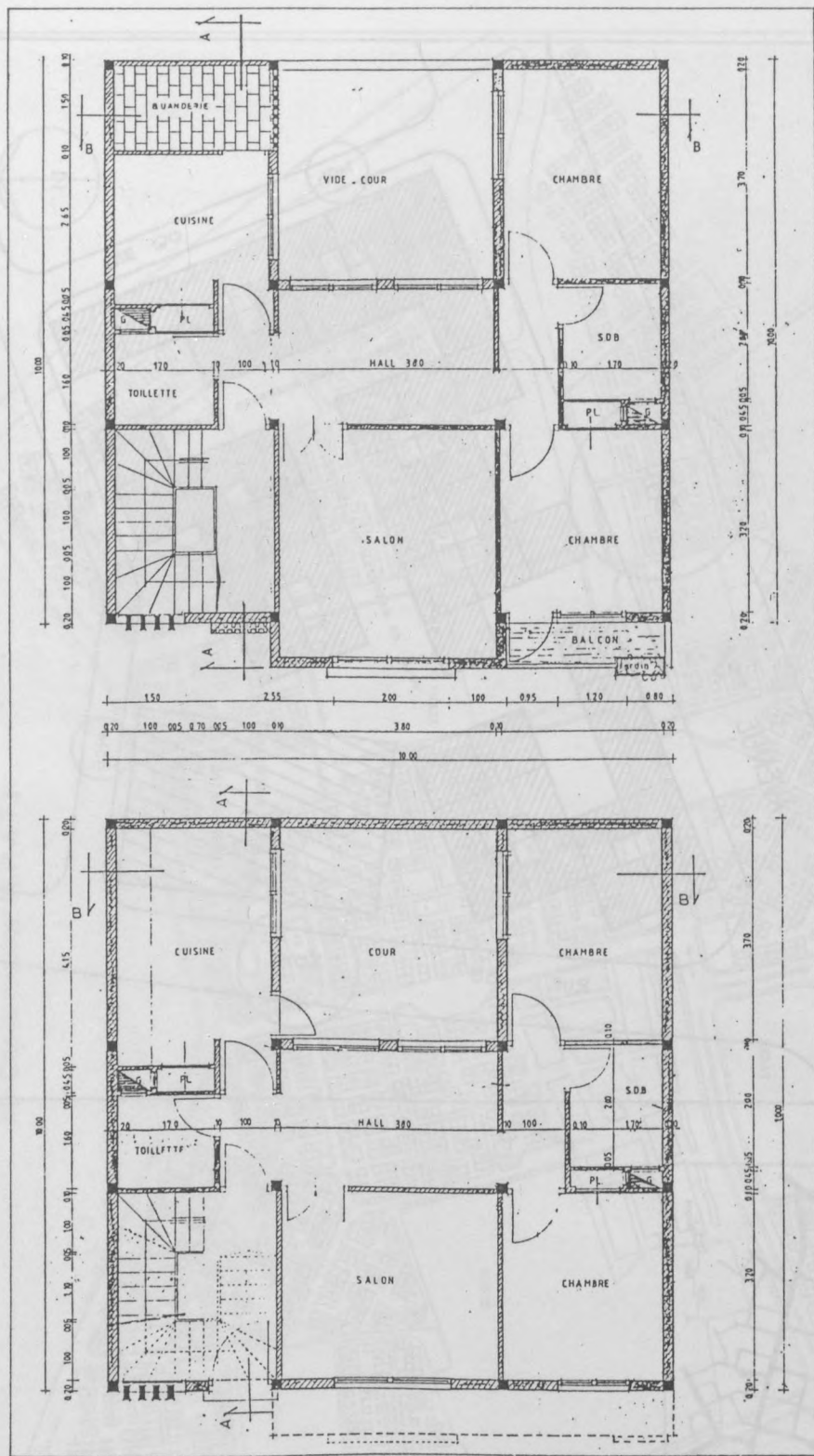
Fig. 7 Plan-type d'immeuble pour le lotissement d'habitat économique Aïn Chock (source: M.H.A.T.)
