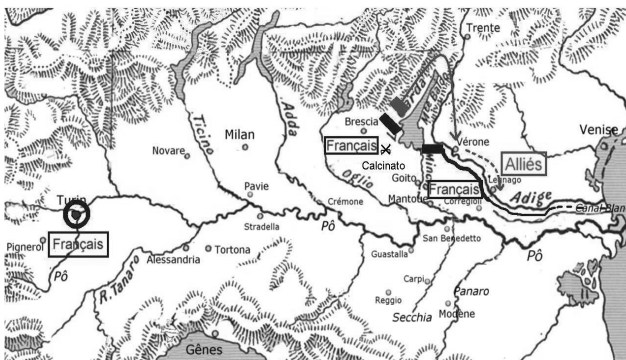
Fig. 1 – Situation générale de l'Italie du Nord après Calcinato, fin mai 1706
