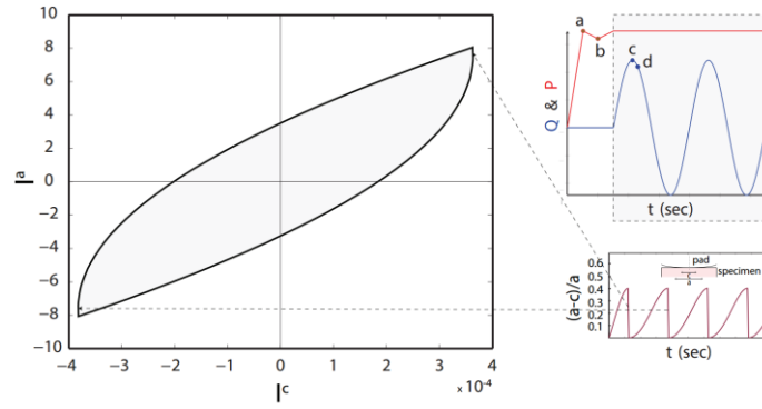
Figure 3: Evolution I^c/I^a sur un cycle de chargement
