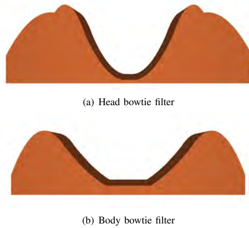
Fig. 6. PENGEOM 3D bowtie filter visualisation.
