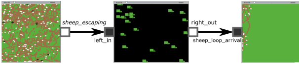
Figure 5: Connexions entre les modèles pour le couplage spatial.
