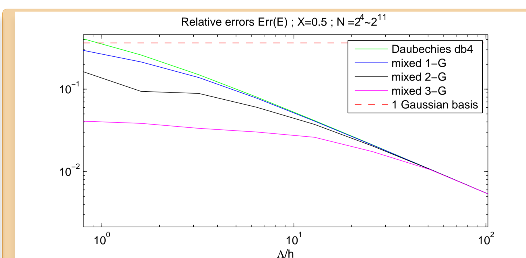
Erreur sur l'énergie en base mixte db4 et CG_{\sigma, X}
