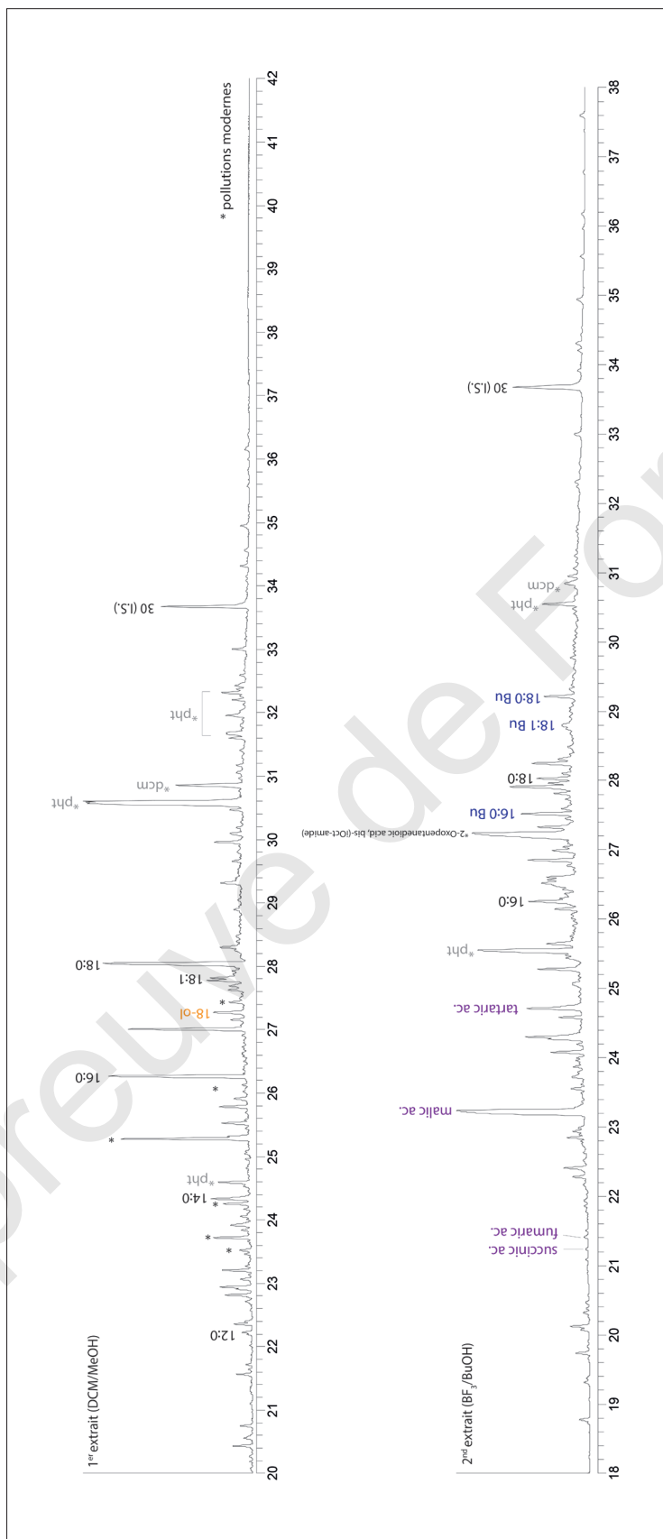
Fig. 4. Chromatogrammes des premiers et seconds extraits obtenus à partir des imprégnations des parois internes de l'amphore n° 4921 (extraits triméthylsilylés, colonne Zebron 5MSi: 20 m x 0.18 mm d.i. x 0.1 µm ép. phase, détecteur MS EI 70 eV). Nicolas Garnier.
