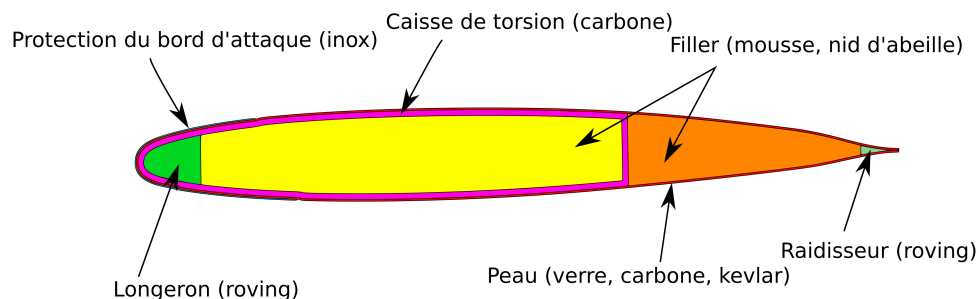
FIGURE 3 – Architecture interne d'une pale de CROR.
