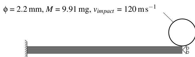
FIGURE 5 – Description de l'essai d'impact transversale sur un toron.
