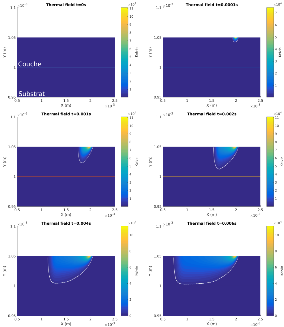
FIGURE 8 – Champ thermique pour une couche d’épaisseur 50\mu\text{m} .
