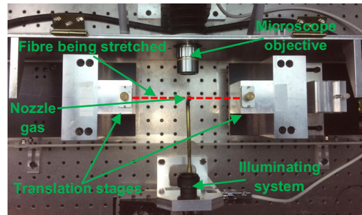
Fig. 1. Pulling rig.
