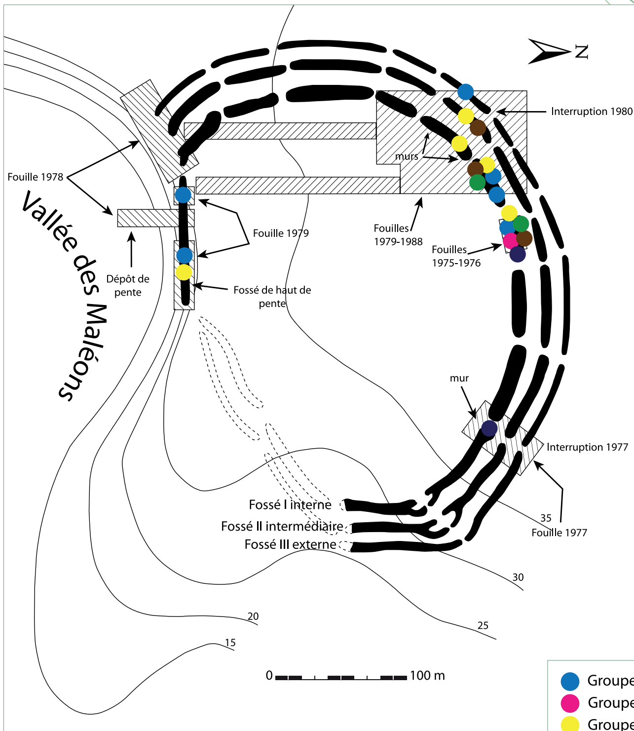
Fig. 469a : Plan de répartition des vestiges de terre crue brûlés dans le comblement des fossés de l'enceinte (DAO : T. Taraud, F. Chanson).
