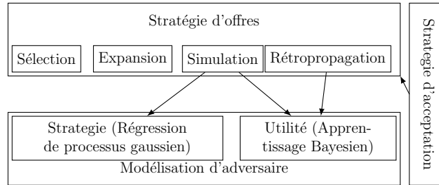
FIGURE 1 – Interaction entre les modules de MoCaNA
