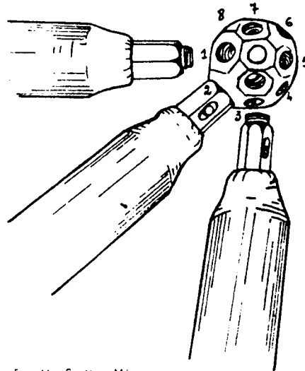
Fig. 41 Système Méro
