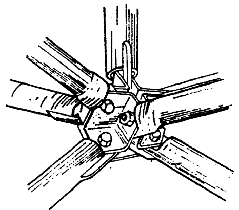
Fig. 43 - Système Varitec
