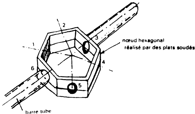
Fig. 42 Système Wupperman
