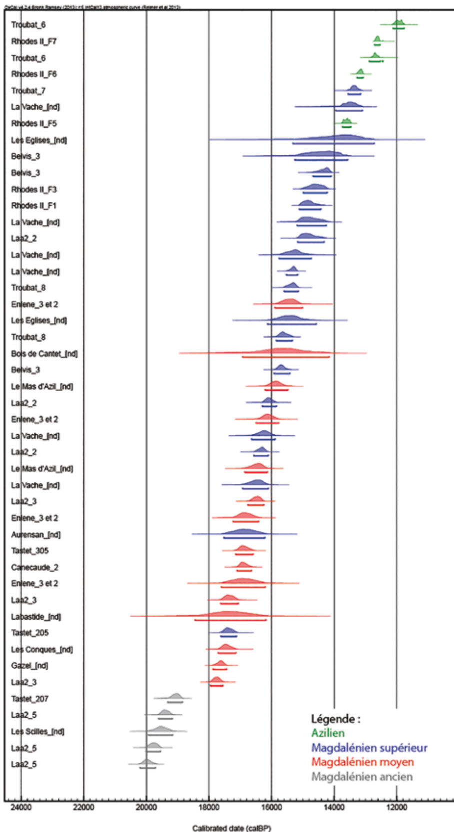
Fig. 2. Les datations radiocarbones (pour le détail des dates, voir tableau 1) / Radiocarbon data (show Table 1 for details about the datations).
