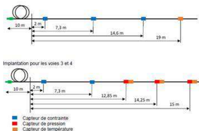
Fig. 6: Position des FBGs le long de la fibre.
