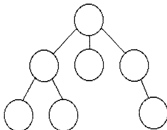
Hiérarchie d'entités
