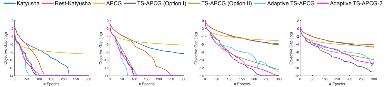
(b) \lambda = 1 \times 10^{-3} , \|x^*\|_0 = 126 (c) \lambda = 5 \times 10^{-4} , \|x^*\|_0 = 618 (d) \lambda = 2 \times 10^{-4} , \|x^*\|_0 = 1250 (e) \lambda = 1 \times 10^{-4} , \|x^*\|_0 = 1594
