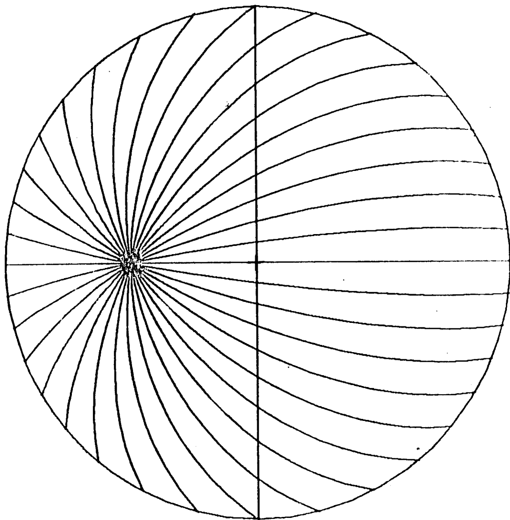
Abaque de traçé de droites parallèles fuyant en un point faisant un angle de 45^\circ avec l'axe de vue.
