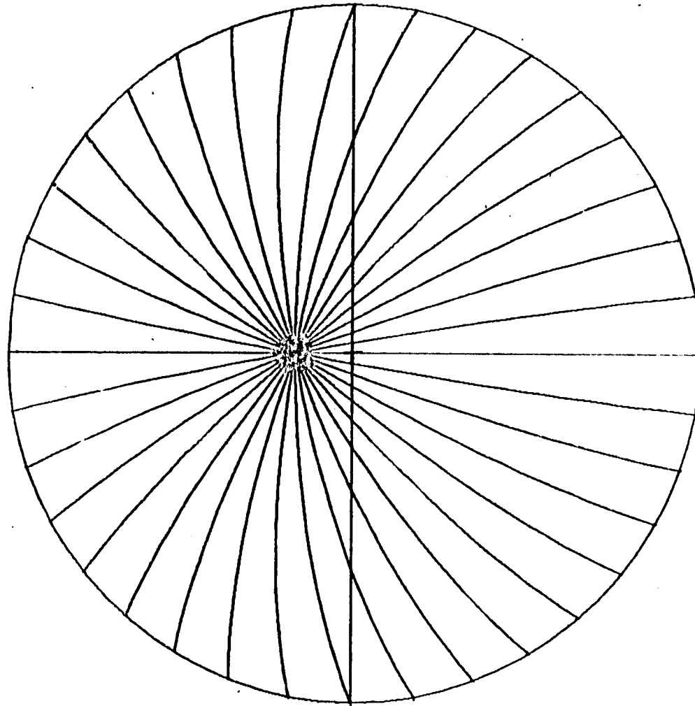
Abaque de traçé de droites parallèles fuyant en un point faisant un angle de 15^\circ avec l'axe de vue.
