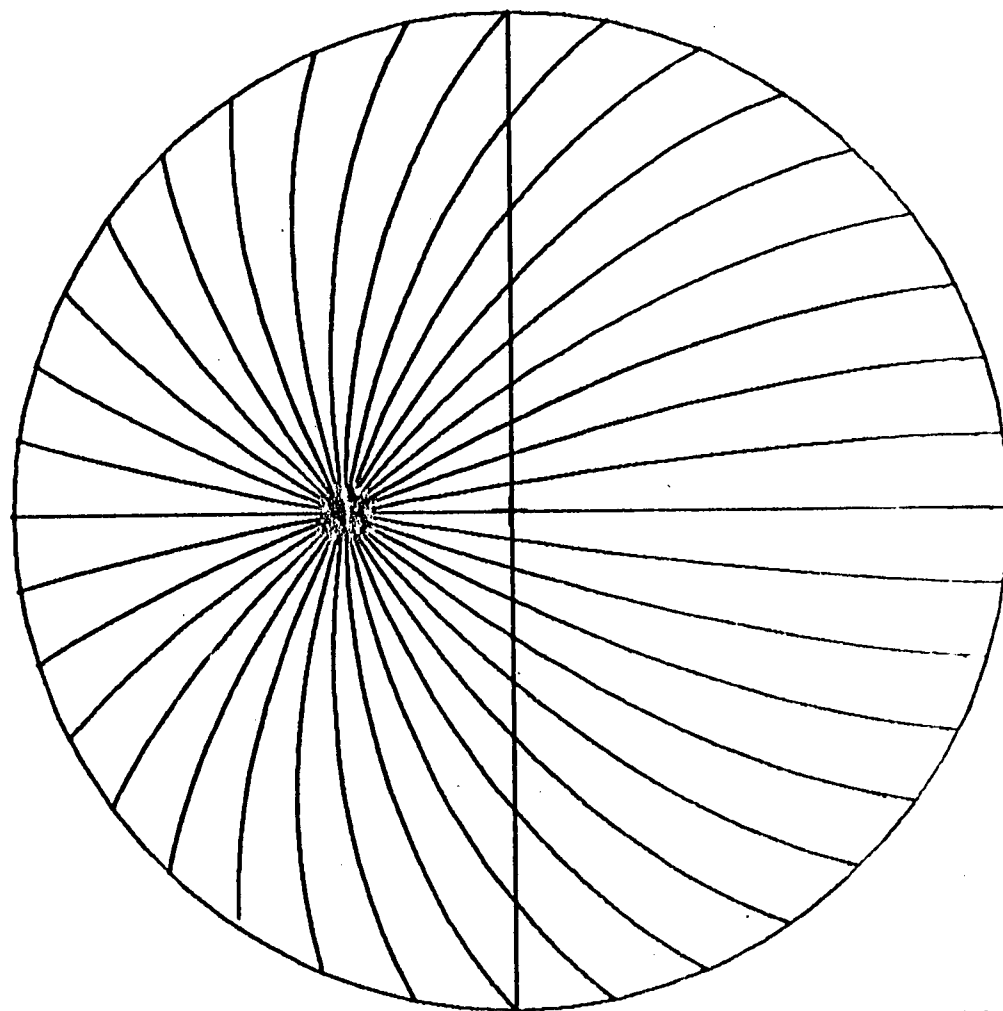
Abaque de traçé de droites parallèles fuyant en un point faisant un angle de 30^\circ avec l'axe de vue.
