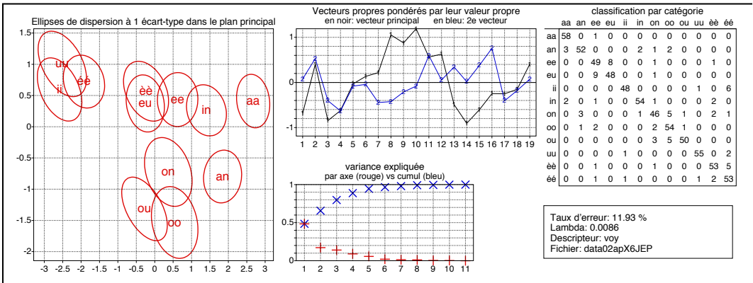
FIGURE 1 – Analyse Discriminante appliquée à la classification des 12 voyelles (9 orales et 3 nasales) du corpus CRC
