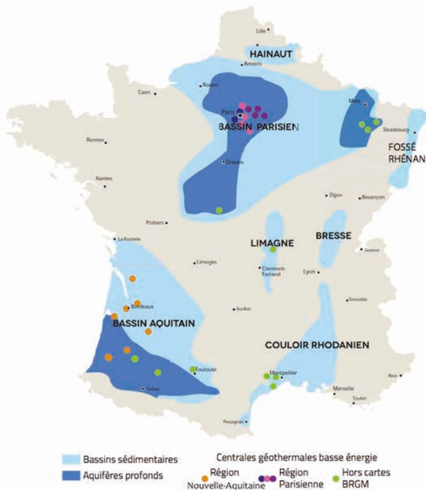
Figure 13 : Installations de géothermie de basse énergie dans les bassins sédimentaires français (modifié d'après le BRGM et l'AFPG) – AFPG (39).
