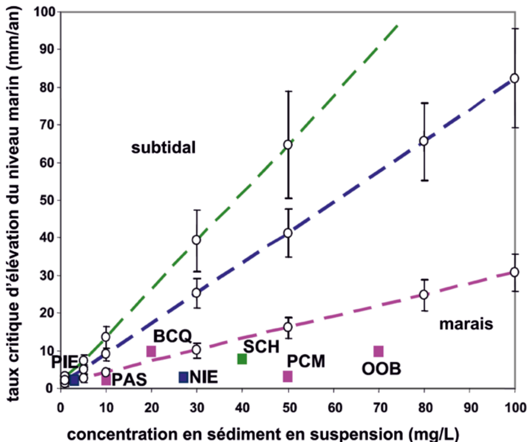
Figure 9 : Limites théoriques de stabilité des marais estuariens et de leur remplacement par des zones subtidales en fonction du taux de remontée du niveau marin et de l'apport sédimentaire, exprimé par la concentration en sédiment en suspension. Lignes verte, bleue et rose : marnage de 5 m, 3 m et 1 m respectivement. Les carrés en couleur représentent des marais estuariens mondiaux avec différentes combinaisons de taux historiques de remontée du niveau marin, marnage et concentration en sédiments en suspension. D'après Kirwan et al. (40).
