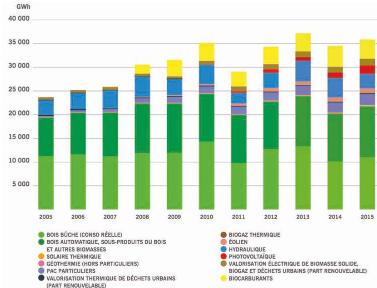
Figure 9 : Évolution de la production énergétique renouvelable (source : AREC (9)).
