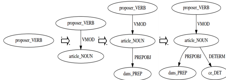
Figure 4 : Extraction de l'ALR <proposer+dans+ce+article>
