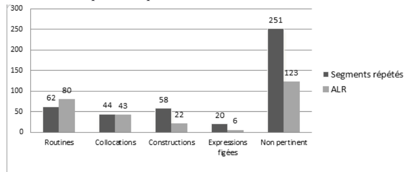
Figure 5 : Comparaison des résultats par type (résultats bruts)
