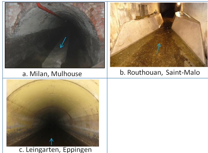
Figure 5 Photos de 3 des 5 sites grandeur nature
