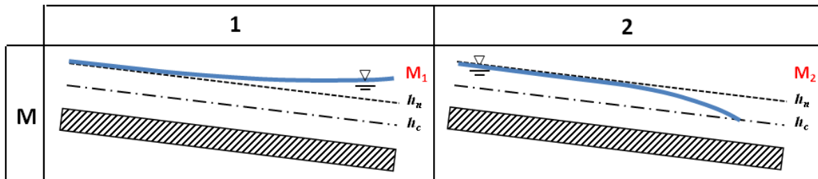
Figure 8 Schéma de courbes de remous de type M (pente faible avec influence (M1) et sans influence (M2))
