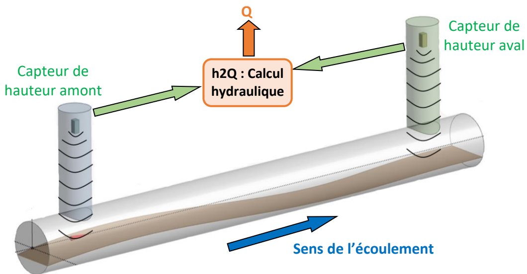
Figure 3 Principe de mesure de la méthode h2Q
