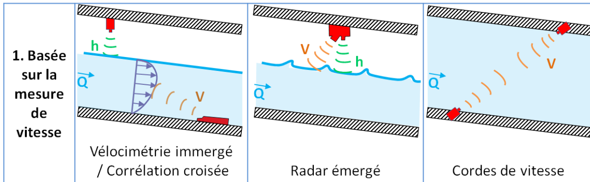
Figure 1 Schéma des différentes technologies d'évaluation du débit avec une mesure de hauteur-vitesse
