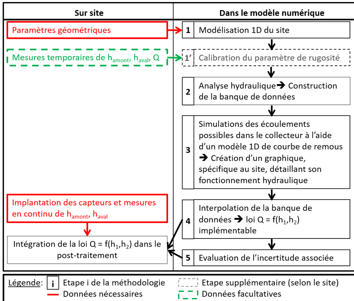
Figure 4 Procédure de mise en application de la méthode
