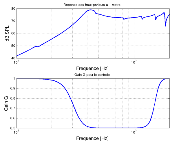
FIGURE 9 – Réponse à 1 m des haut-parleurs montés sur la sourdine (haut) ; gain G appliqué au contrôle (bas) avec G_0 = 0,5 , fréquences de coupure f_1 = 300 \text{ Hz} et f_2 = 1500 \text{ Hz} , paramètres de la sigmoïde \lambda_1 = \frac{10}{f_1} et \lambda_2 = \frac{20}{f_2}
