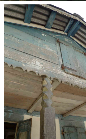
Planches de rive, dont la forme découpée réduit la pression du vent dans la galerie et en dessous de la toiture.
