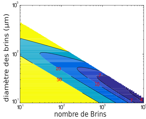
Fig. 10. Résistance AC des fils de LitZ par rapport au cas où toute la fenêtre est remplie de cuivre
