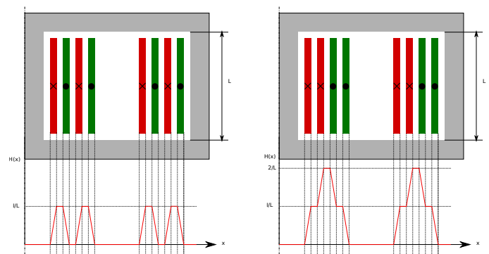
Fig. 13. Composante verticale de H_{fuite} dans la fenêtre de bobinage selon la manière dont sont intercalés les feuillards. Il y a deux spires au primaire et au secondaire séparées en deux blocs
