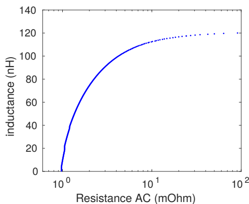
Fig. 11. Évolution de l'inductance de fuite avec la résistance AC lorsque l'épaisseur d'isolant varie de 10 μm à 3.29 mm. On observe le cas qui minimise R_{ac} pour chaque épaisseur d'isolant.
