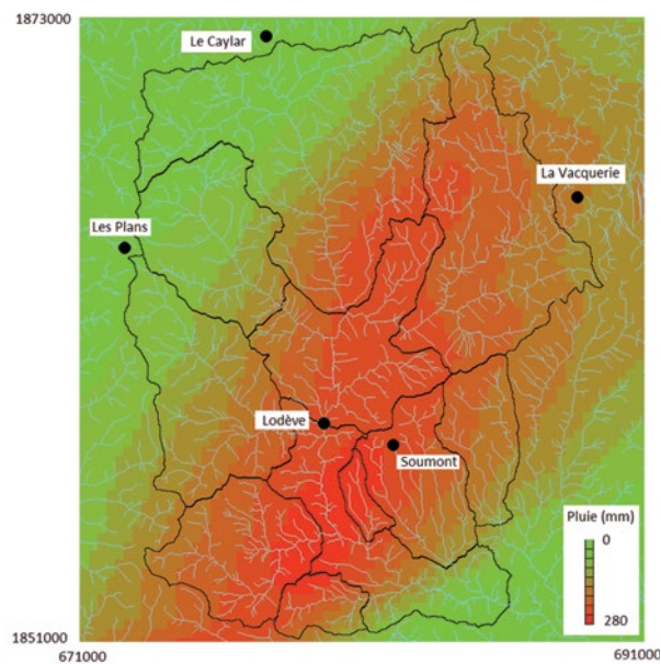
Figure 3 : Répartition spatiale des cumuls de pluie sur 3h, de 15h à 18h TU le 12/09/2015, d’après les données Panthère Météo-France
