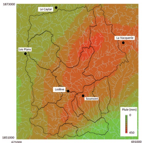
Figure 2 : Répartition spatiale des cumuls de pluie sur 12h 12/09/15 14 :00 TU au 13/09/15 02 :00 TU sur les sous-bassins de la Lergue d’après les données Panthère Météo-France
