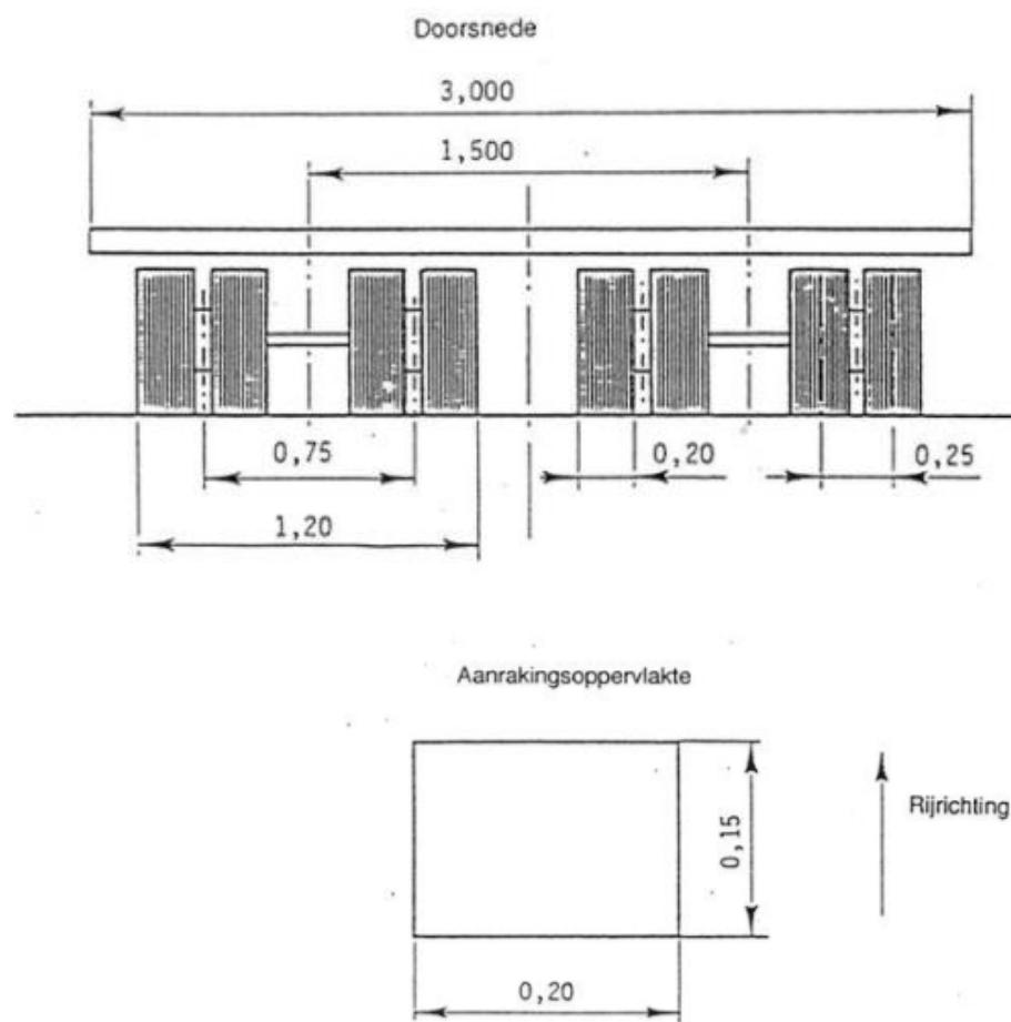
Afb. 3 - Belastingsschema 2
