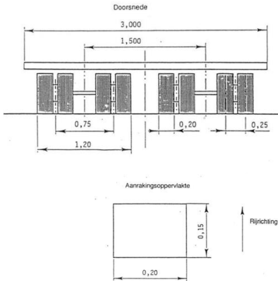
Afb. 3 - Belastingsschema 2
