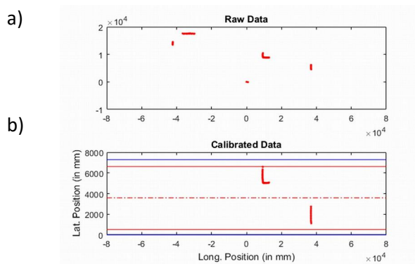
Figure 12 : Données LiDAR brutes (haut) - Données LiDAR calibrées (bas); ligne bleu: bord de plateforme, ligne rouge: marquages de rive, ligne pointillée: marquage d'axe
