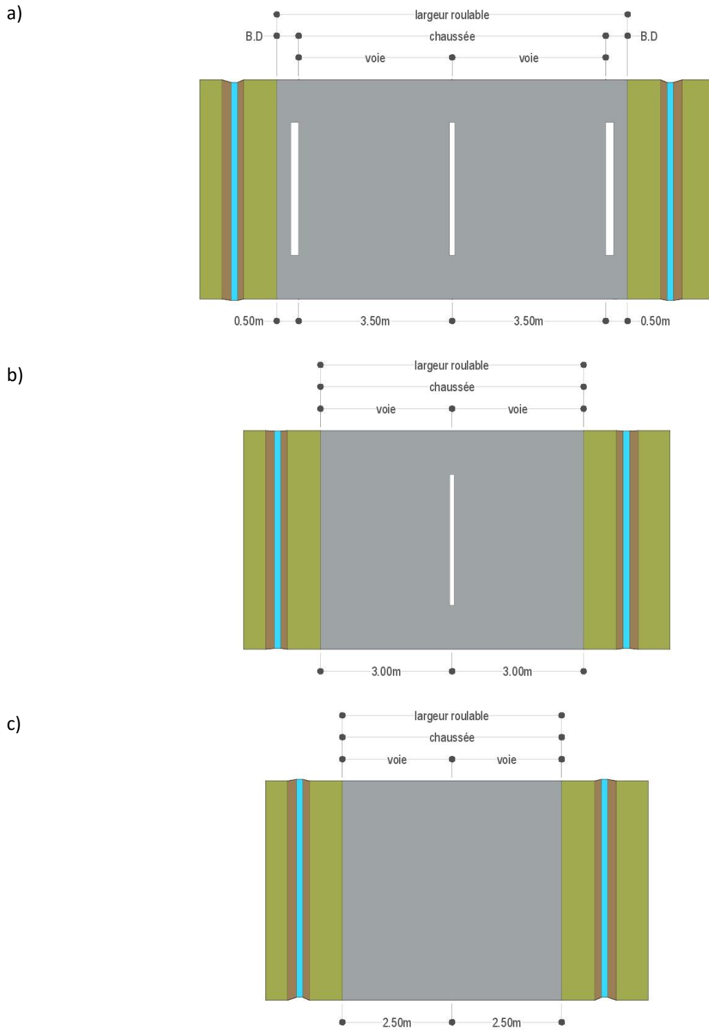
Figure 21 : Les principales caractéristiques des profils en travers des routes bidirectionnelles : a) cas d'une chaussée avec marques d'axe et de rives ; b) cas d'une chaussée avec marques d'axe uniquement ; c) cas d'une chaussée sans marques sur chaussée. B.D : Bande dérasée.
