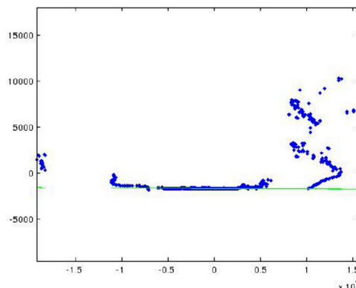
Figure 9 : Profil en travers mono-déversé : a) Caméra de scène ; b) Nuage de points (en bleu) et estimation du dévers (en vert).
