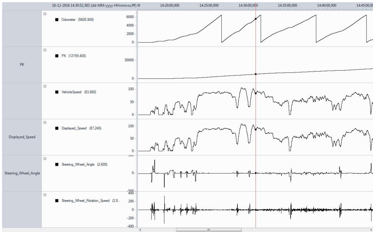
Figure 25 : Exemple de données issues du bus CAN visualisées dans le logiciel The Observer XT.
