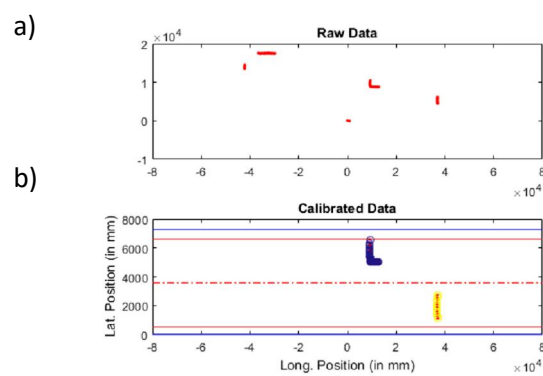
Figure 13 : Données LiDAR brutes (haut) - Données LiDAR calibrées avec détection des véhicules (bas)
