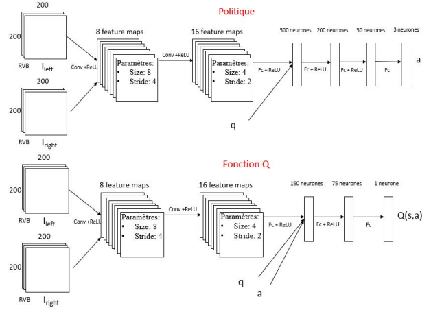
FIGURE 3 – Structure de la politique et de la fonction Q -vaieur
