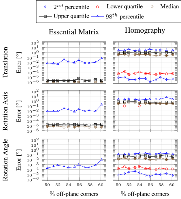
FIGURE 4 – Erreurs obtenues lorsque le calibrage est parfait et les points donnés en coordonnées entières
