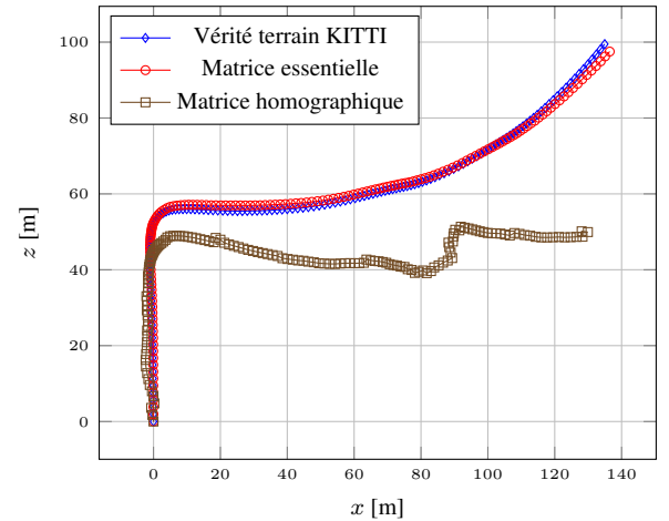
FIGURE 8 – Trajectoires obtenues sur la séquence 03 de KITTI jusqu’à l’image 150
