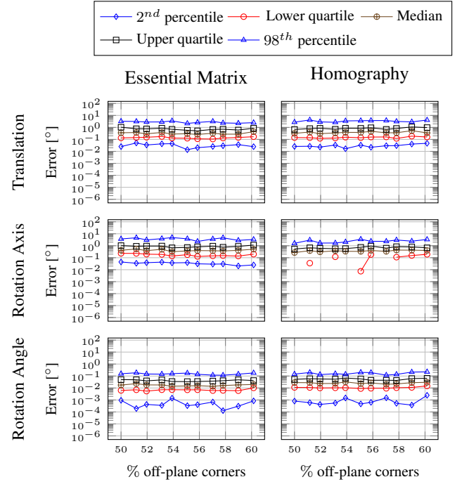
FIGURE 5 – Erreurs obtenues lorsque le calibrage est parfait et les points donnés en coordonnées entières
