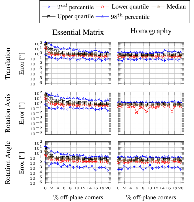
FIGURE 7 – Erreurs obtenues lorsque le calibrage est perturbé par \mathcal{N}(0, 100) et les points donnés en coordonnées entières
