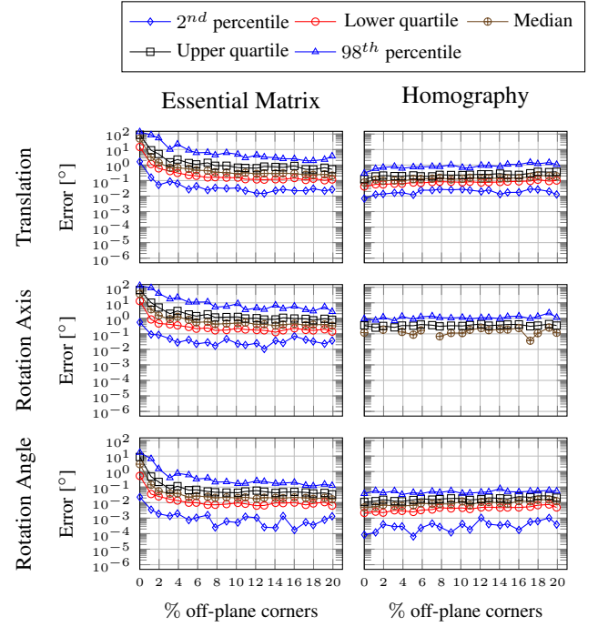
FIGURE 3 – Erreurs obtenues lorsque le calibrage est parfait et les points donnés en coordonnées entières
