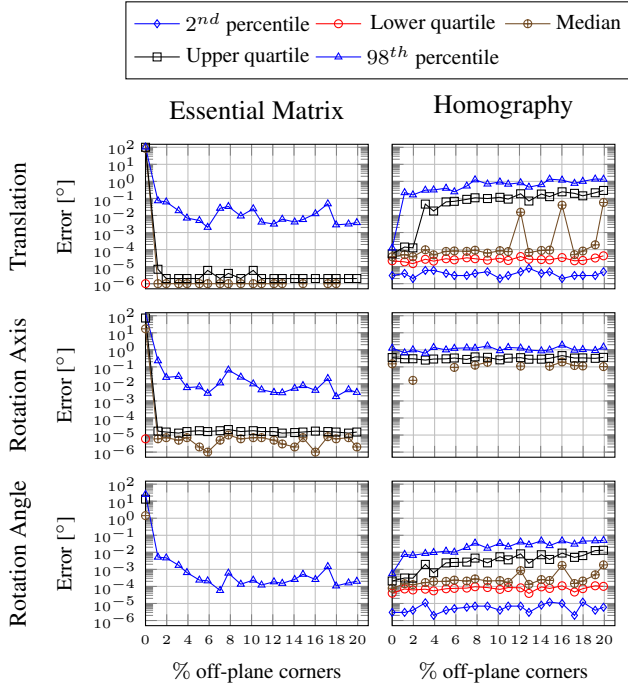
FIGURE 2 – Erreurs obtenues lorsque le calibrage est parfait et les points donnés en coordonnées flottantes
