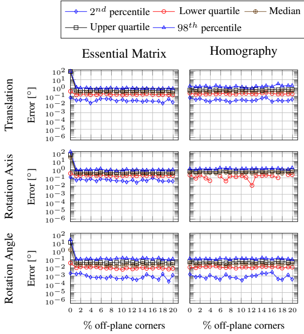
FIGURE 6 – Erreurs obtenues lorsque le calibrage est perturbé par \mathcal{N}(0, 100) et les points donnés en coordonnées flottantes
