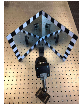
FIGURE 1 – Système Stéréo Catadioptrique multi-Plan composé d'une caméra et deux miroirs plans
