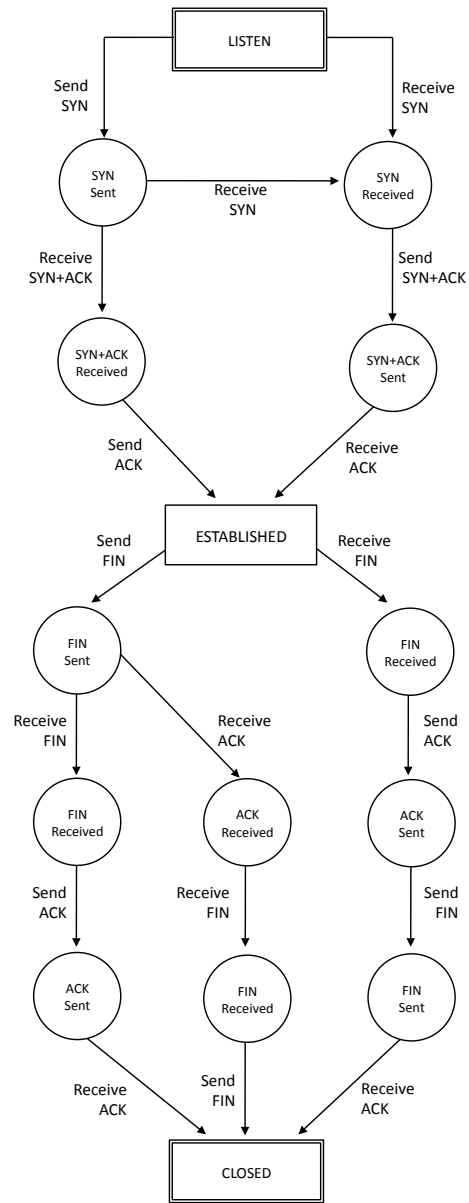
FIG. 1. Automate d'états pour TCP.
