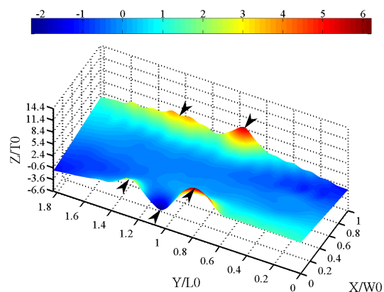
Fig. 15: DIC : point 4
