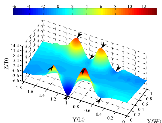
Fig. 19: DIC : point 6
