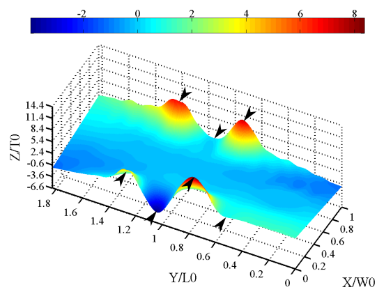
Fig. 17: DIC : point 5
