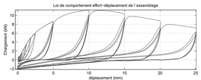
Les essais permettent d'établir les lois de comportement effort-déplacement et ainsi d'estimer l'énergie dissipée par la structure.
