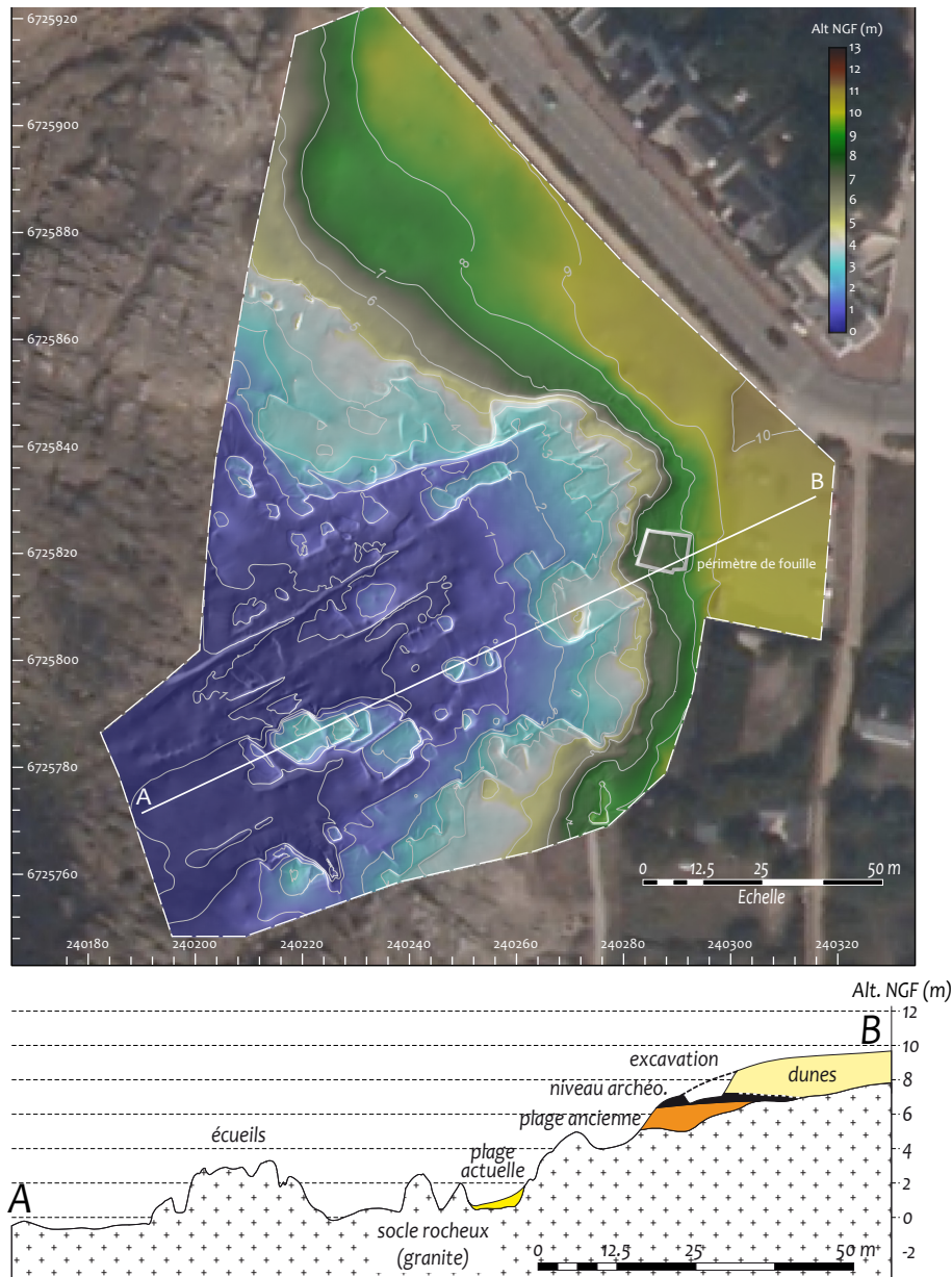
Fig. 9 – Modèle numérique de terrain (MNT) réalisé à proximité du site archéologique de Beg-er-Vil représentant le modelé topographique de l'estran. Ici, le MNT est superposé à l'orthophotographie littorale prise le 28 septembre 2011 à 10 h 40 (UTM; source : ©Ortho Littorale V2 – MEDDE). Un profil topographique a été extrait du MNT entre les points A et B (DAO P. Stéphan).
