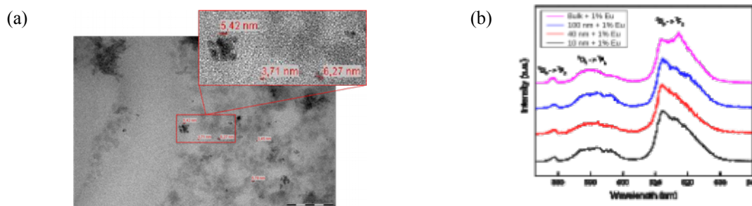
Fig. 1. a. TEM images of Eu-doped silica nanoparticles (~10 nm diameter) b. Emission spectra of 1% Eu-doped silica bulk and nanoparticles of various diameters (cette figure ne me semble pas de très bonne résolution. Parce que j'ouvre un .doc avec open office ?)
